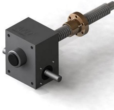
SPINDELHUBGETRIEBE - R
